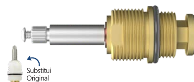
012501 TORNEIRA DOCOL COMPLETO
