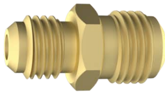
170700 Amarelo Rosca Externa: TC 1/2" NIPLE DE REDUÇÃO 1/2" X 3/8" Rosca Externa: TC 3/8" Material: Latão
