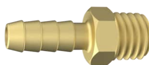
170502 | Saída Externa: TM 1/4" 170503 | Saída Externa: TM 5/16"
