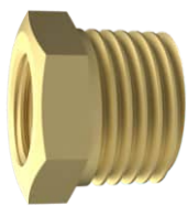
170600 | Rosca Interna: NPT 1/8" 170601 | Rosca Interna: NPT 1/4" 170602 | Rosca Interna: NPT 3/8" BUCHA DE REDUÇÃO NPT X TM Rosca Externa: NPT 1/2" Acabamento: Amarelo Material: Latão
