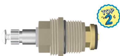
018500 TORNEIRA E DUCHA HIGIÊNICA IDEAL METAIS
