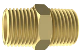
171100 | Rosca Externa: NPT 1/8" 171102 | Rosca Externa: NPT 1/4" 171103 | Rosca Externa: NPT 3/8" 171104 | Rosca Externa: NPT 1/2" NIPLE NPT Acabamento: Amarelo Material: Latão
