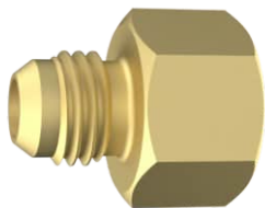
170900 Amarelo Rosca Externa: TC 3/8" TERMINAL BSP X TC Rosca Interna: BSP 1/2" Material: Latão
