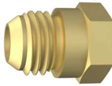
171150 | Rosca Interna: NPT 1/8" 171151 | Rosca Interna: NPT 1/4" UNIÃO REDUTORA TC X NPT Rosca Externa: TC 3/8" Acabamento: Amarelo Material: Latão
