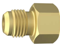
170901 Amarelo Rosca Externa: TC 1/2" TERMINAL BSP X TC Rosca Interna: BSP 3/8" Material: Latão
