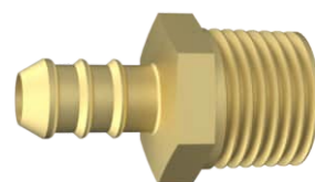
170501 | Saída Externa: TM 3/8" 170504 | Saída Externa: TM 5/16" 170505 | Saída Externa: TM 1/2"
